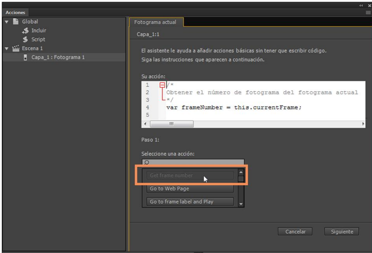
Captura de pantalla de muestra con opciones del asistente de código de acciones
