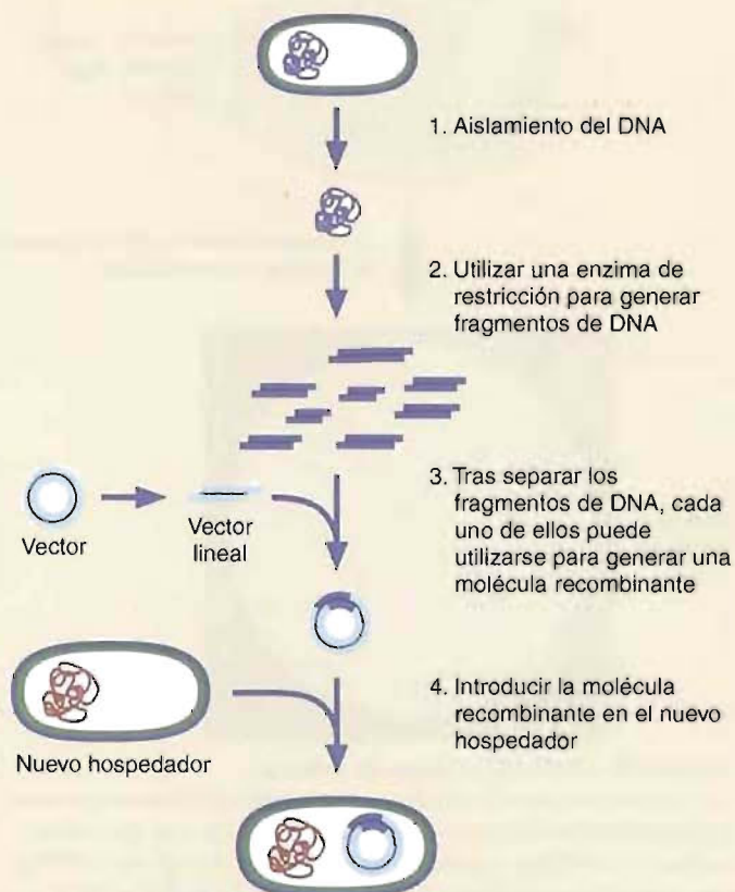
FIGURA 18B Clonación del DNA.
