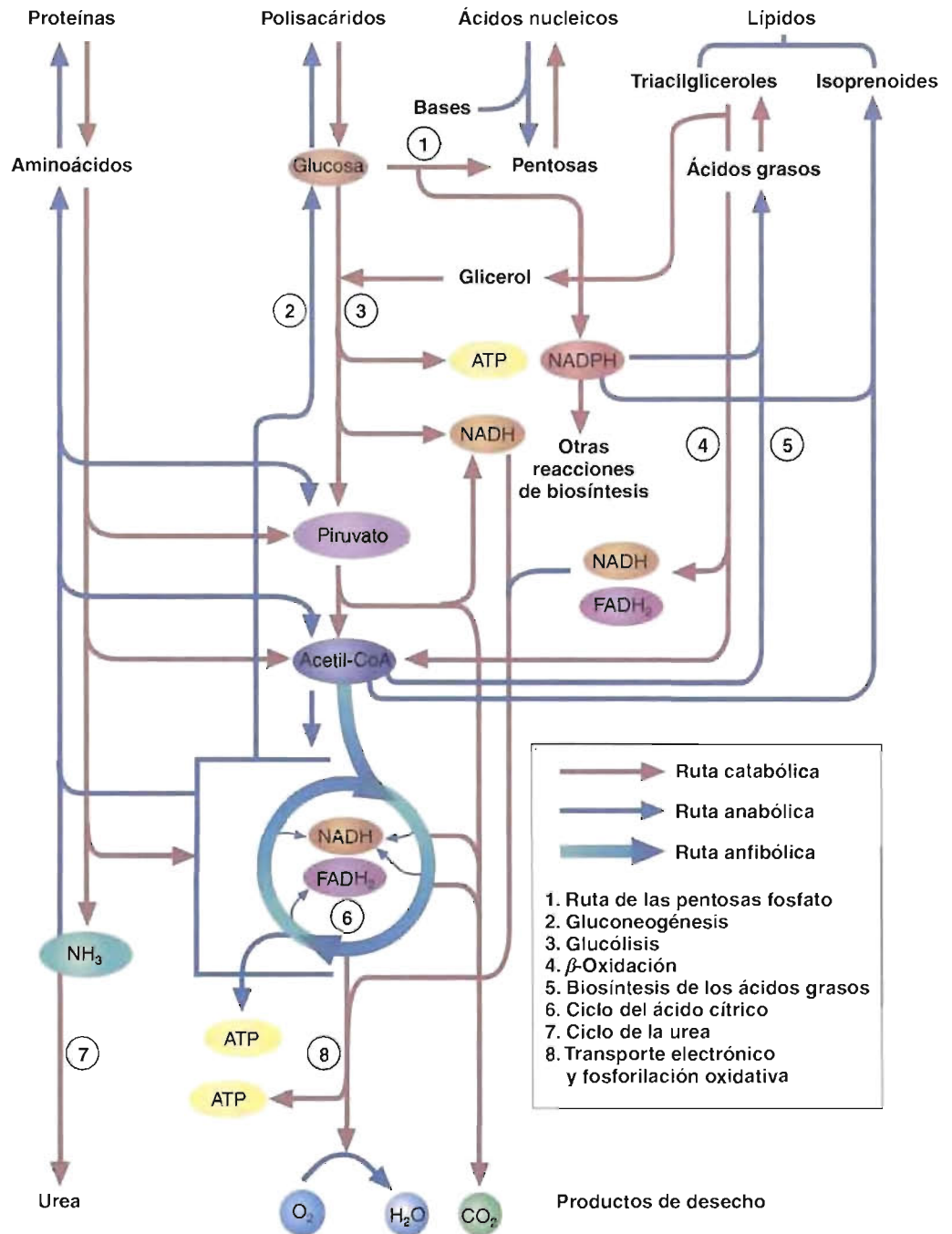
FIGURA 16-1 Visión general del metabolismo. En esta visión general simplificada del metabolismo, se presentan las rutas anabólicas y catabólicas de las principales moléculas de alimento de los heterótrofos (es decir, aquellas rutas bioquímicas que sintetizan, degradan o interconvierten biomoléculas importantes y generan energía).
