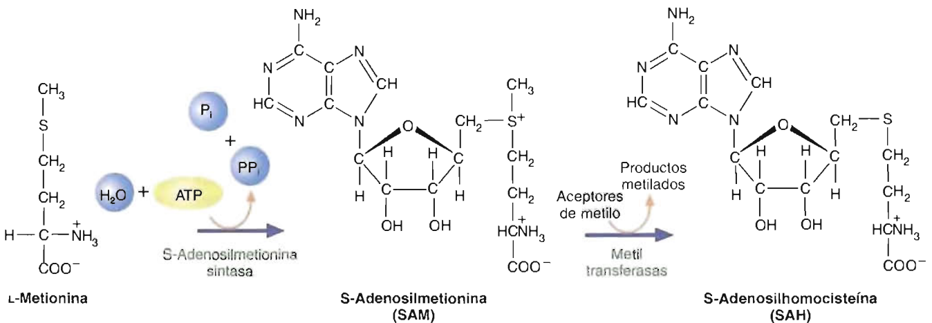
FIGURA 14-16 Formación de S-adenosilmetionina.
