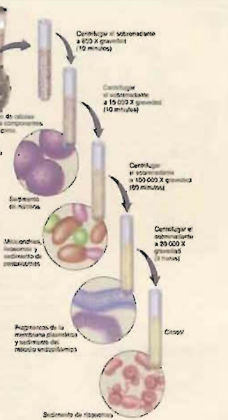
FIGURA 2D Fraccionamiento celular. Tras la homogeneización de las células en un líquido, se separan los componentes celulares en una serie de centrifugaciones, a velocidades cada vez mayores. Al añadir cada centrifugación, se separa el sedimento, se coloca en un tubo nuevo de centrifugación y se vuelve de nuevo a una velocidad centrifugación mayor. El sobrenadante restante puede reutilizarse en otro líquido y observarse por microscopía en un tubo de centrifugación.
