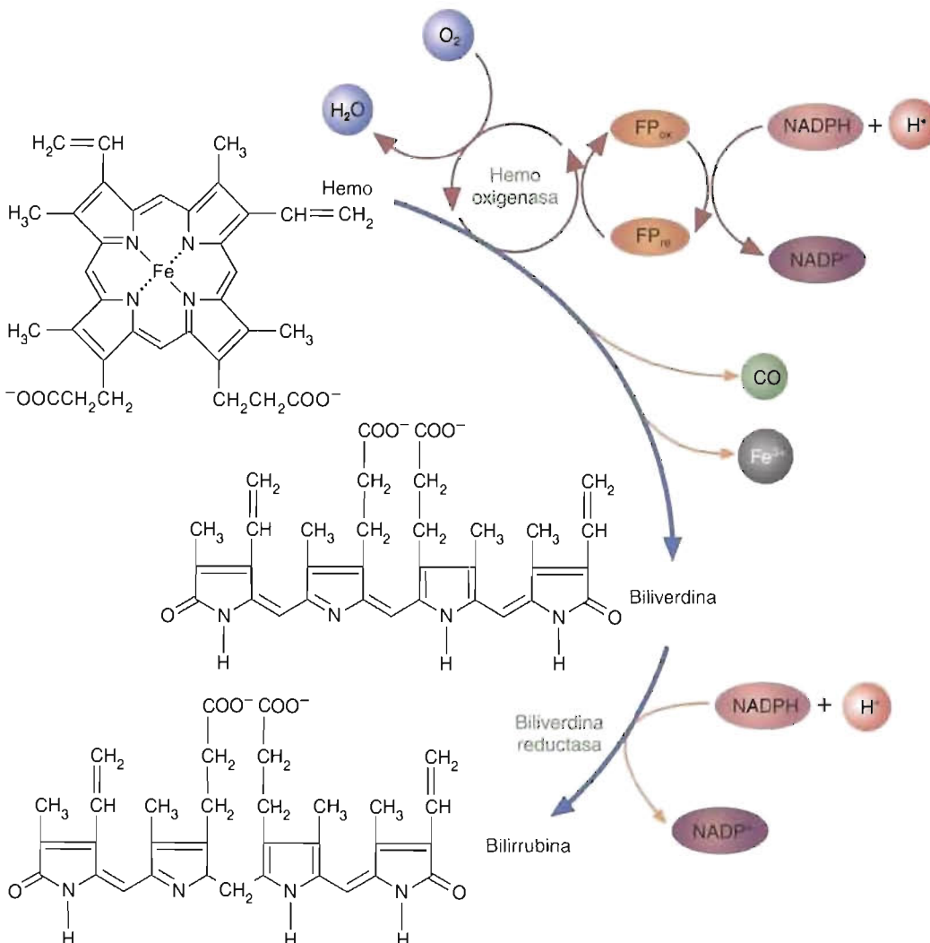
FIGURA 15-15 Síntesis de bilirrubina.
