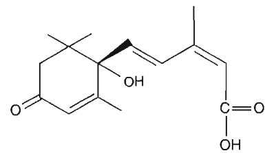
Ácido abscísico (regulador del crecimiento vegetal)
