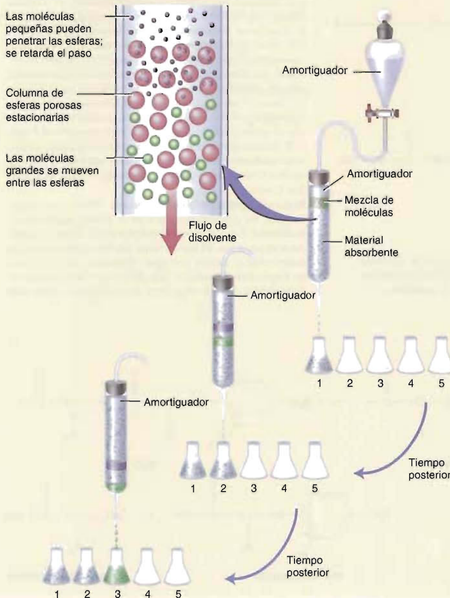
FIGURA 5C Cromatografía de filtración en geles
