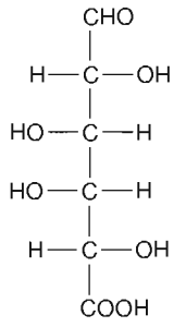
Ácido urónico
