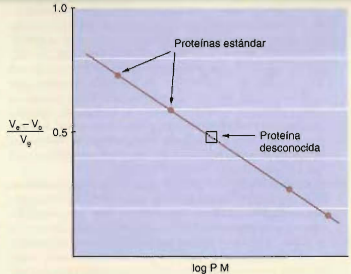
FIGURA 5D Determinación del peso molecular utilizando cromatografía de filtración en geles.
