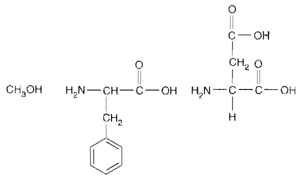
Metanol Fenilalanina Ácido aspártico
