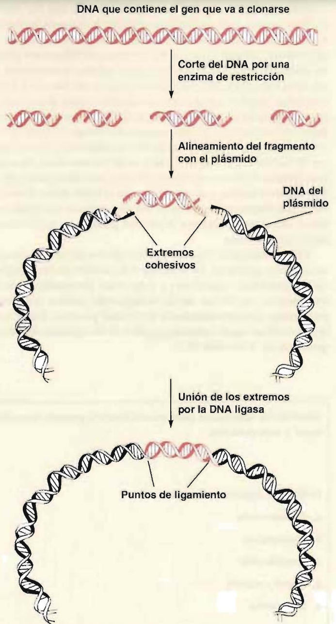
FIGURA 18A Construcción de un DNA recombinante.
