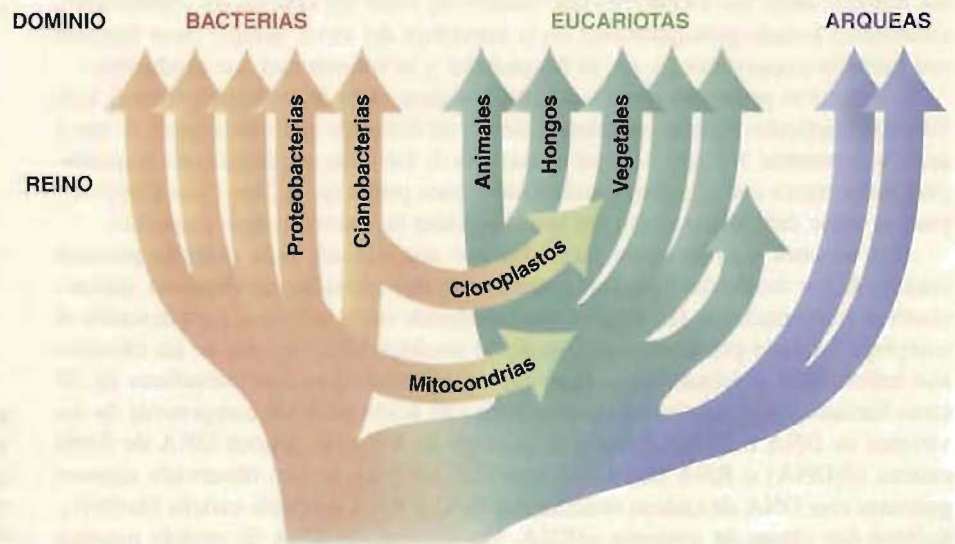
FIGURA 17I Modelo actual del árbol de la vida. El diagrama simplificado, que ilustra las relaciones filogenéticas entre los organismos actuales, se basa en el grado de semejanza de las secuencias de RNA ribosómico. Los procesos endosimbióticos que han generado los cloroplastos y las mitocondrias se indican por las flechas diagonales superior e inferior.
