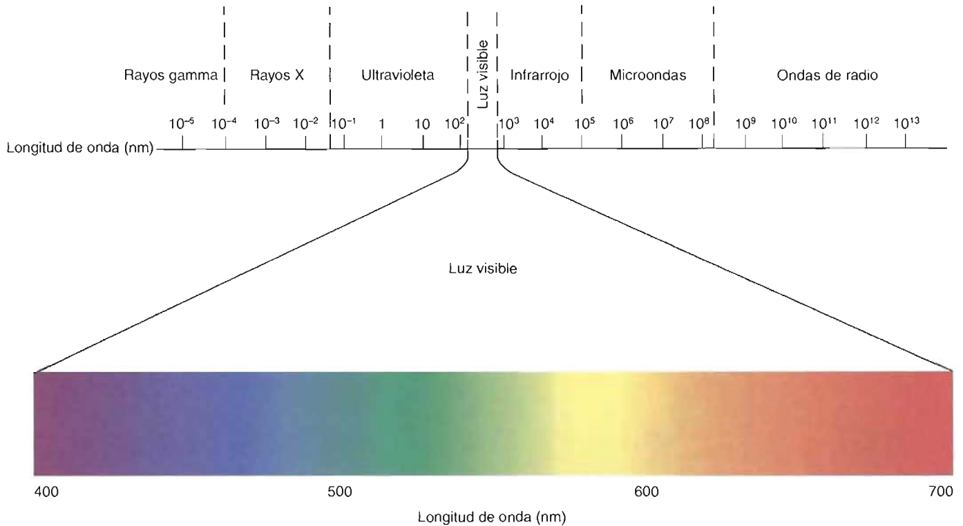
FIGURA 13-5 Espectro electromagnético.
