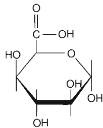
Ácido \alpha -D-idurónico
