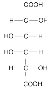
Ácido aldárico
