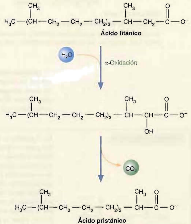
FIGURA 12C \alpha -Oxidación del ácido fitánico.
