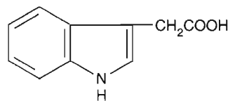
Auxina (ácido indol acético)
