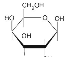
\beta -D-Galactosa
