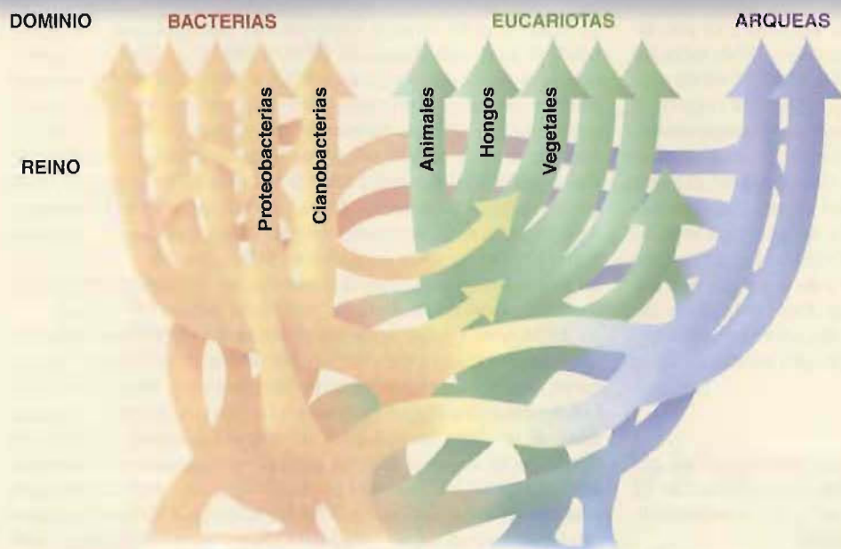
FIGURA 17J Árbol (o «red») de la vida modificado que se ha propuesto.
