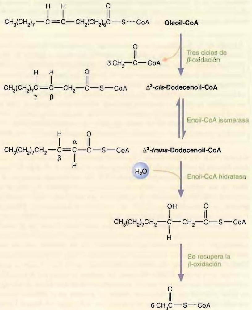
FIGURA 12A \beta -Oxidación de la oleoil-CoA.
