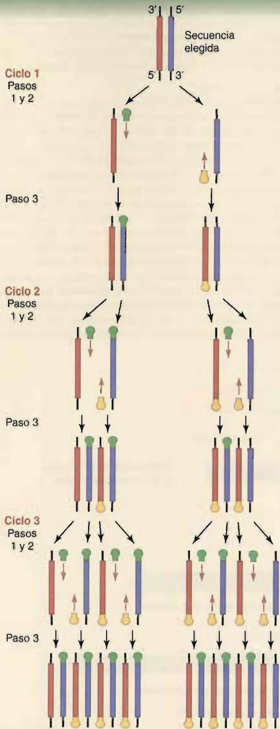
FIGURA 1BE Reacción en cadena de la polimerasa. Una única molécula de DNA puede amplificarse millones de veces repitiendo un ciclo de tres pasos. En el primer paso, el dsDNA de la muestra se desnaturaliza por calentamiento a 95 °C. En el paso 2 se baja rápidamente la temperatura hasta 50 °C y se añade un oligonucleótido cebador. El cebador hibrida con las secuencias complementarias de los extremos de las dos cadenas. Durante el paso 3, se produce la síntesis de DNA al aumentar la temperatura hasta 70 °C, la temperatura óptima de la polimerasa Taq. Se repite luego el ciclo en el que actúan como moldes las cadenas viejas y las nuevas.
