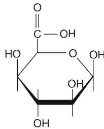
Ácido \beta -D-idurónico
