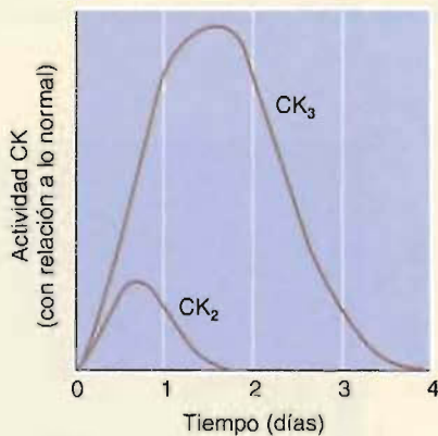
FIGURA 6B Patrón característico de las concentraciones en suero de la creatina quinasa tras un infarto de miocardio.
