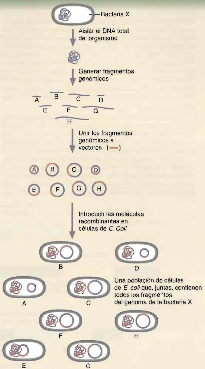
FIGURA 1BF Creación de una biblioteca de DNA utilizando el método de escopetazo. Tras aislar el DNA del organismo y purificarlo, se fragmenta con una enzima de restricción. Los fragmentos se incorporan aleatoriamente en vectores y las moléculas recombinantes se introducen en células como E. coli . La colección de estas células se denomina biblioteca genómica.
