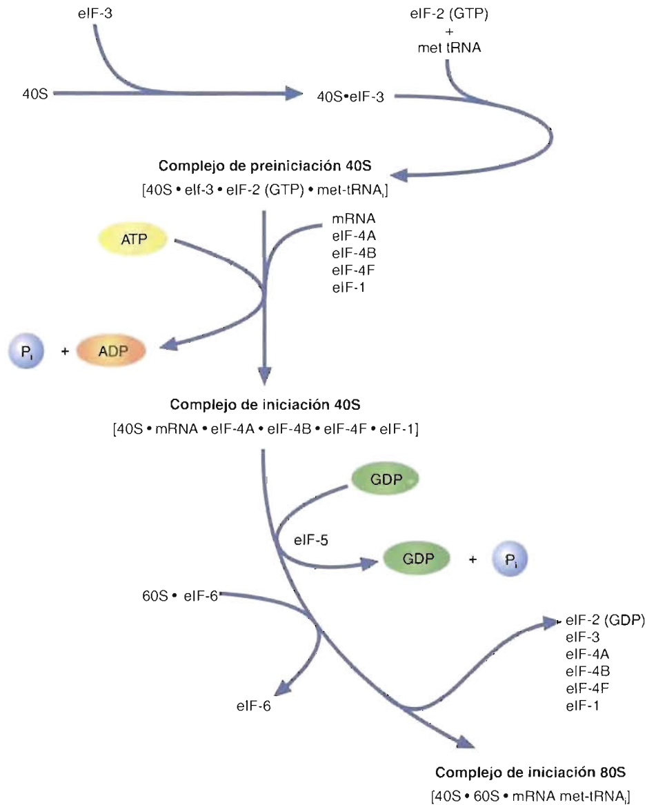
FIGURA 19-10 Formación del complejo de iniciación en los eucariotas.
