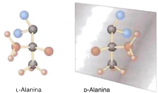
L-Alanina
