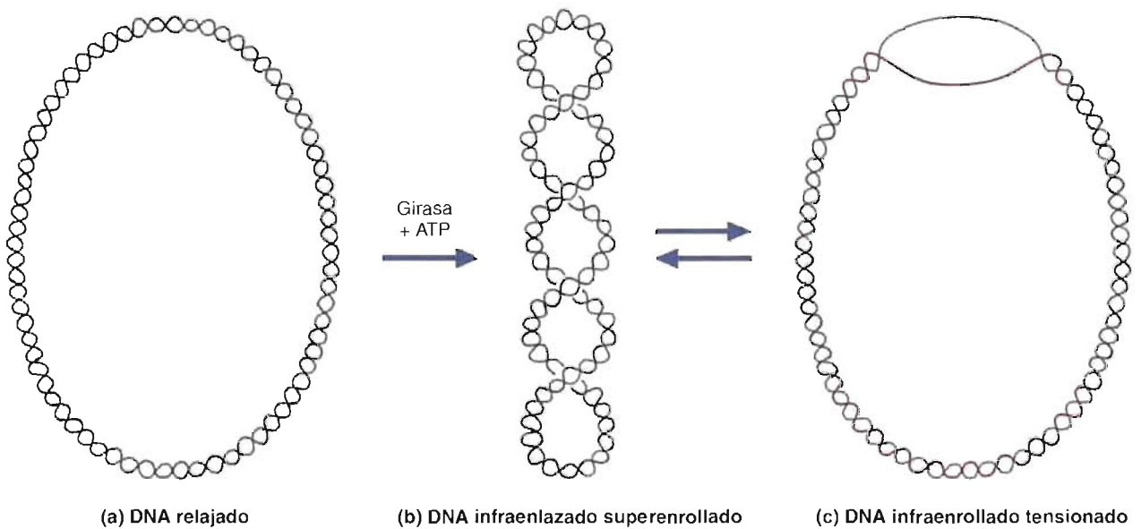
(a) DNA relajado
