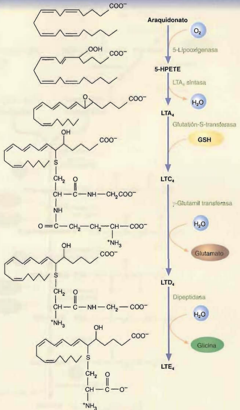
FIGURA 12E Síntesis de leucotrienos seleccionados.
