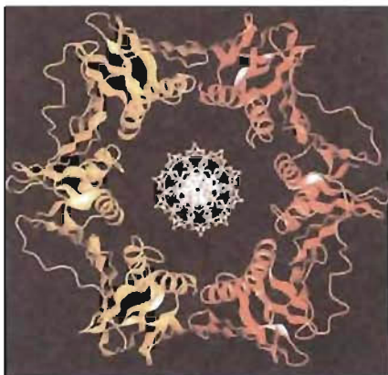
FIGURA 18-4 Corte transversal de la subunidad \beta de la DNA polimerasa III.
