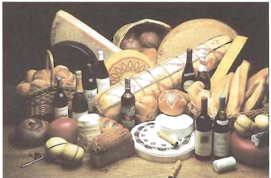
Productos de la fermentación. Los seres humanos utilizan determinados microorganismos para metabolizar los azúcares en ausencia de oxígeno y producir queso, vino y pan.
