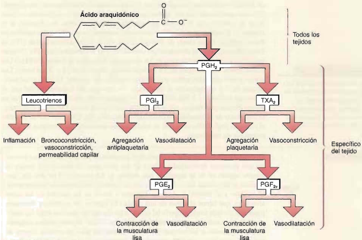
FIGURA 11B Acciones biológicas de moléculas de eicosanoides seleccionadas. En el Capítulo 12 se considera la síntesis de estas moléculas.
