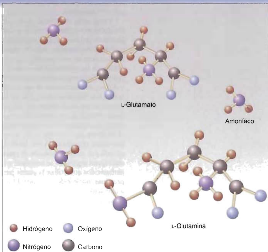
Metabolitos del nitrógeno. El glutamato, la glutamina y el amoníaco se encuentran entre las moléculas más importantes del metabolismo del nitrógeno.
