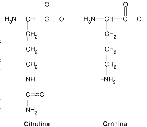
FIGURA 5-6 Citrulina y ornitina.
