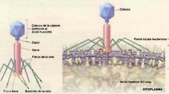
FIGURA 17.26 Bacteriófago T4. (a) El genoma de DNA del bacteriófago T4 induce la síntesis por la célula hospedadora de unas 30 proteínas. (b) Penetración de la pared celular de la célula hospedadora por un bacteriófago.
