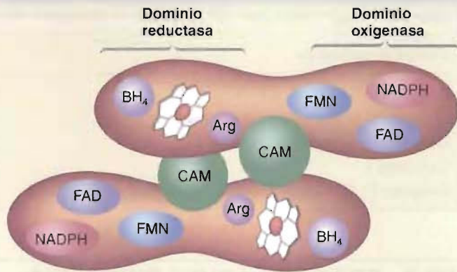
FIGURA 10B Estructura esquemática de la NOS.
