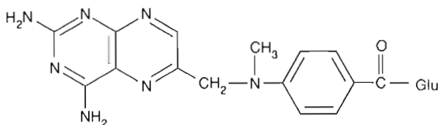
Ametofterina (metotrexato)
