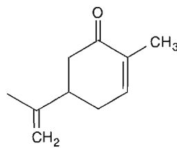
Carvona (aceite de hierbabuena)
