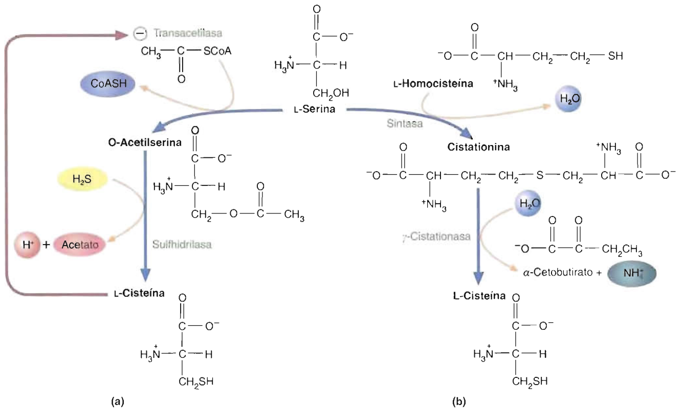
FIGURA 14-7 Biosíntesis de cisteína
