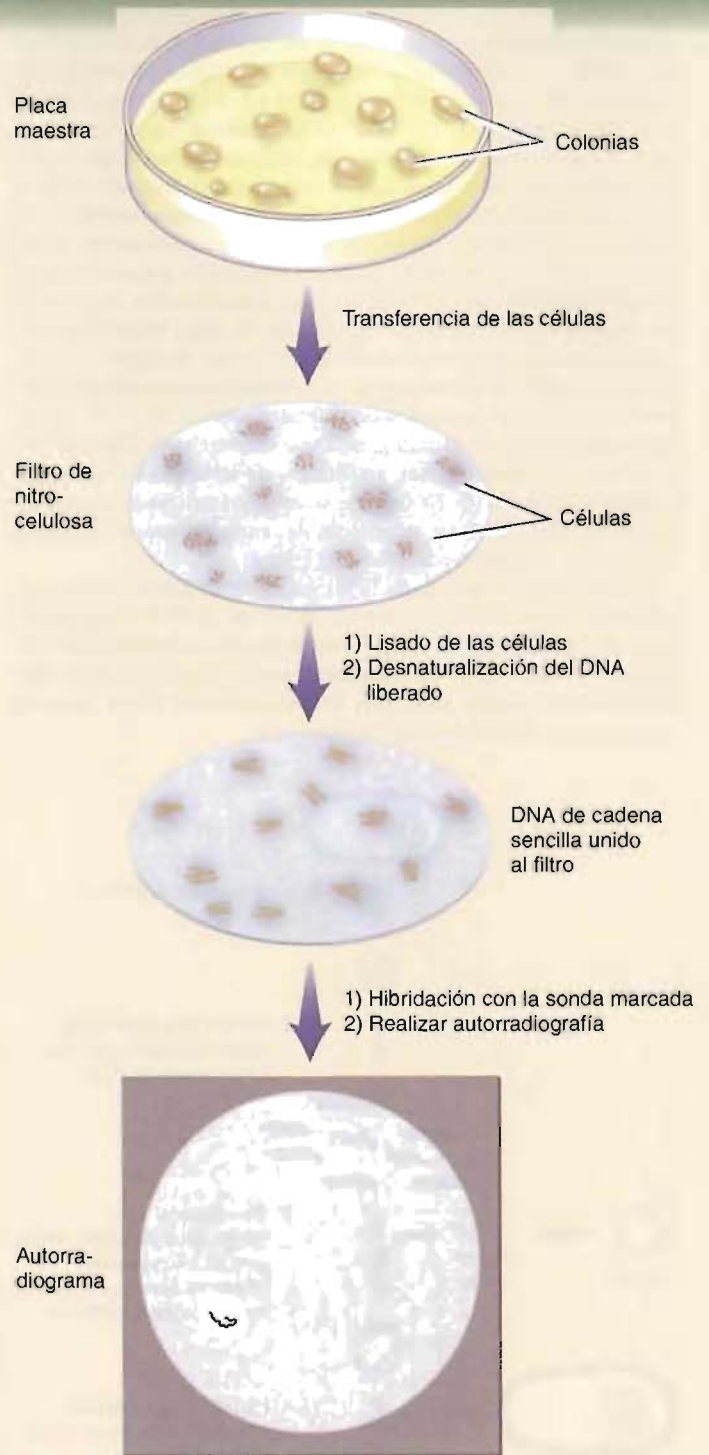
FIGURA 18D Hibridación de colonias. Las células bacterianas se siembran en un medio sólido que sólo permite el crecimiento de las células transformadas. Una vez que las colonias se han hecho visibles, la placa se transfiere a un filtro de nitrocelulosa. Las células que se agarran al filtro se lisan y el DNA que se libera se desnaturaliza y se desproteíniza. Tras añadir una sonda marcada, las moléculas de la sonda que no han hibridado se eliminan mediante lavado. Las células que poseen secuencias de DNA que hibridan con la sonda se identifican comparando el autorradiograma del filtro con un patrón.
