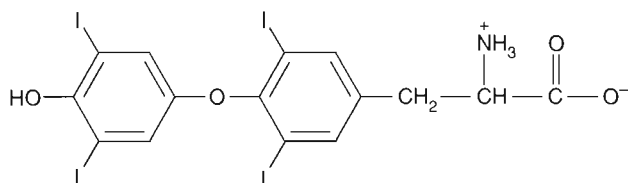
Tiroxina ( T_4 )
