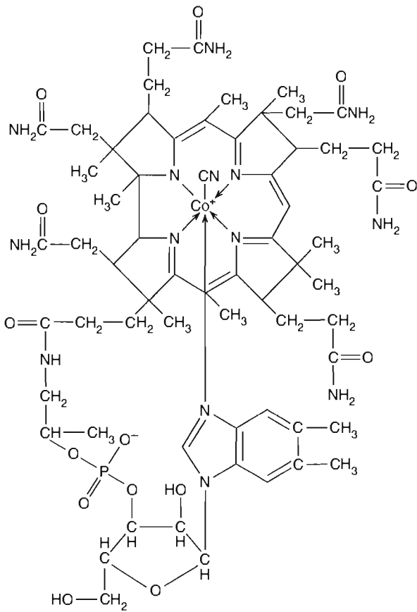
FIGURA 14-15 Estructura de la cianocobalamina, un derivado de la vitamina B 12 .
