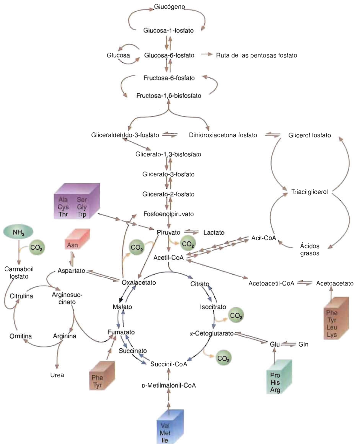
FIGURA 16-3 Metabolismo de los nutrientes en los mamíferos.
