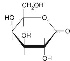
\delta -Lactona del ácido galactónico
