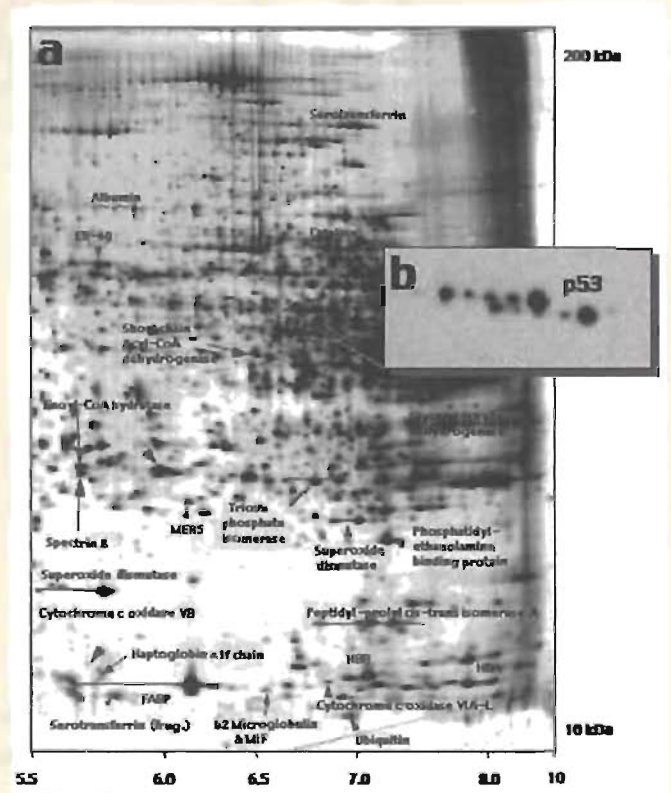
FIGURA 19B Patrón bidimensional en gel. Tras añadir el extracto de hígado al gel, se corre primero en un gradiente de pH (puntos isoeléctricos) y luego en un SDS-PAGE para separar las proteínas de acuerdo con su masa molecular. La inserción muestra un agrandamiento de múltiples versiones de p53, un producto de un protooncogén, que se ha revelado por tratamiento con anticuerpos.
