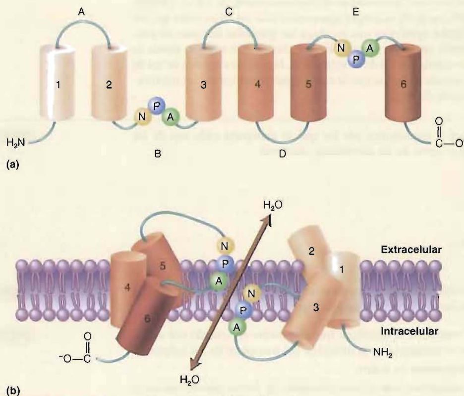
FIGURA 11E Representación esquemática del monómero de acuaporina. Cada monómero de AQP-1 posee seis hélices \alpha que se expanden por la membrana y que están conectadas por cinco bucles (a). En el monómero funcional, los dos bucles que contienen las secuencias NPA forman el lugar selectivo del agua (b).
