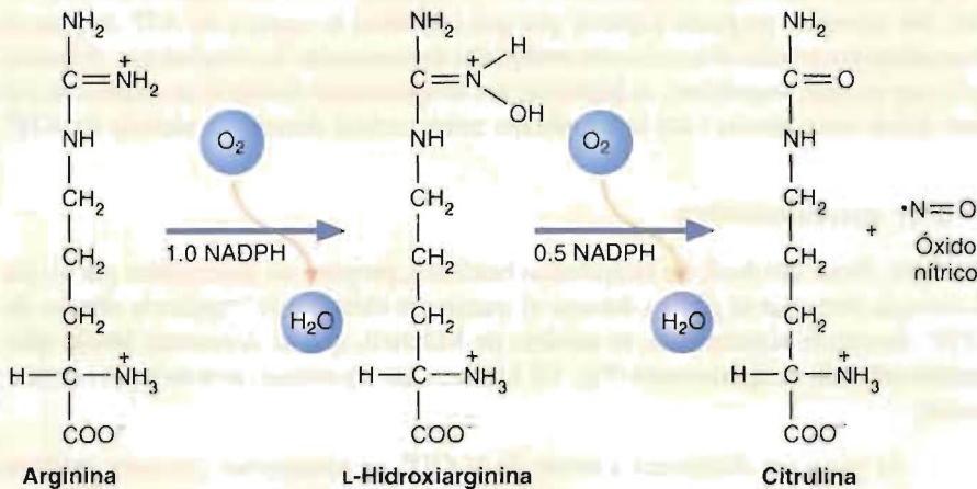
FIGURA 10A Reacción catalizada por la NOS.
