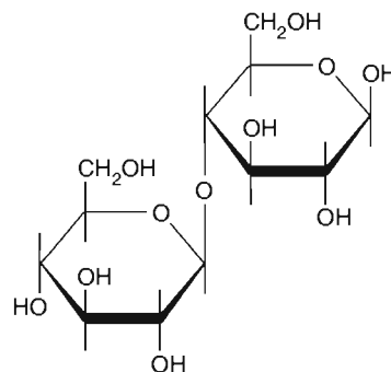
FIGURA 7-28 \beta -Celobiosa.
