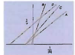
FIGURA 6-12 Representación de Lineweaver-Burk.
