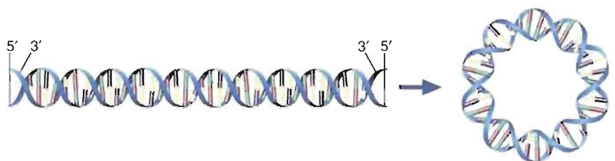
Molécula de DNA lineal de doble cadena
