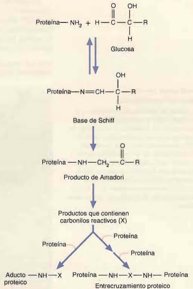
FIGURA 16B Reacción de Maillard.
