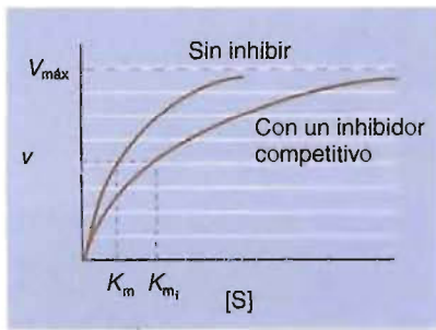
FIGURA 6-8 Representación de Michaelis-Menten de una actividad enzimática sin inhibir frente a una inhibición competitiva.
