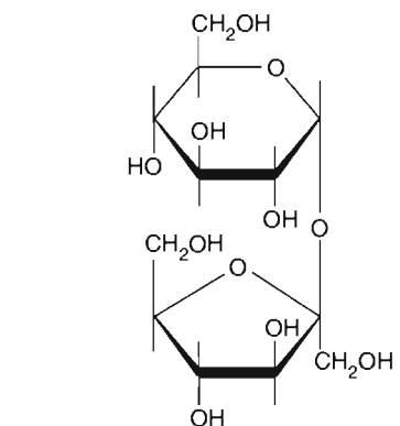
FIGURA 7-29 Sacarosa. Los residuos de glucosa y fructosa están unidos por un enlace glucosídico \alpha, \beta(1,2) .
