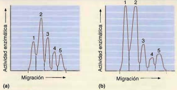
FIGURA 6C Patrón electroforético de las isoenzimas de lactato deshidrogenasa.
