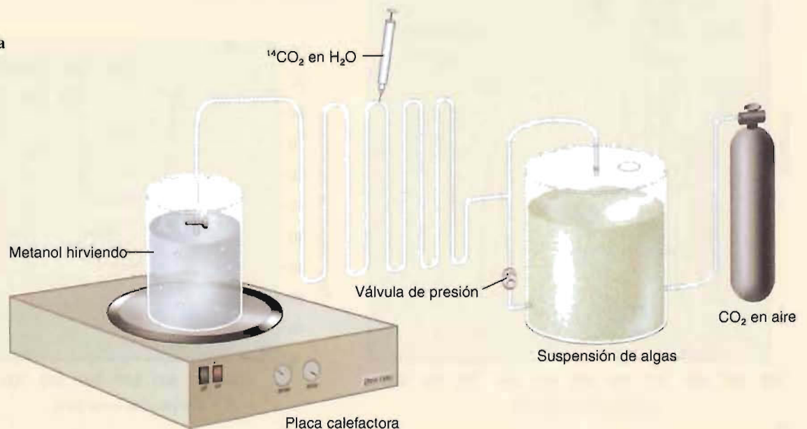
FIGURA 13E Aparato de Calvin para investigar la fijación de CO_2 .
