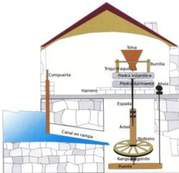
Funcionamiento de un molino hidráulico
