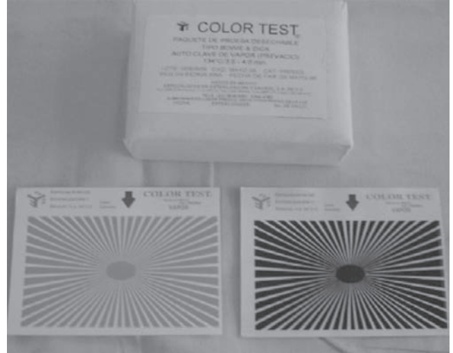
Figura 8-10. Indicadores para vapor saturado.
