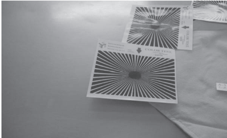
Figura 8-20. Prueba realizada en la esterilización por vapor saturado de prevació. Sirve para constatar que la penetración del vapor en el paquete ha sido rápida y uniforme y que en él no hay aire ni gases no condensables. Se utiliza el paquete de prueba o estándar B&D. En el centro del paquete se encuentra un indicador químico específico. Este indicador tiene impresos, con tinta sensible al vapor, círculos concéntricos o líneas a través de toda su superficie. Se coloca sólo el paquete estándar y en posición horizontal sobre la válvula de drenaje. Se procesa en un ciclo específico para B&D, con un tiempo meseta de esterilización limitado a 3.5 min. Al finalizar el ciclo se valida la homogeneidad en el viraje del indicador; la presencia de aire o gases no condensables se detecta cuando el color de todos los círculos del indicador no ha virado a negro uniforme.
