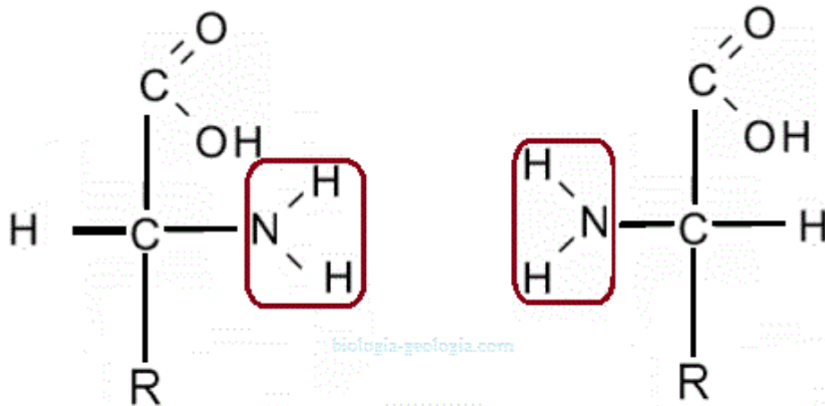
D aminoácido
