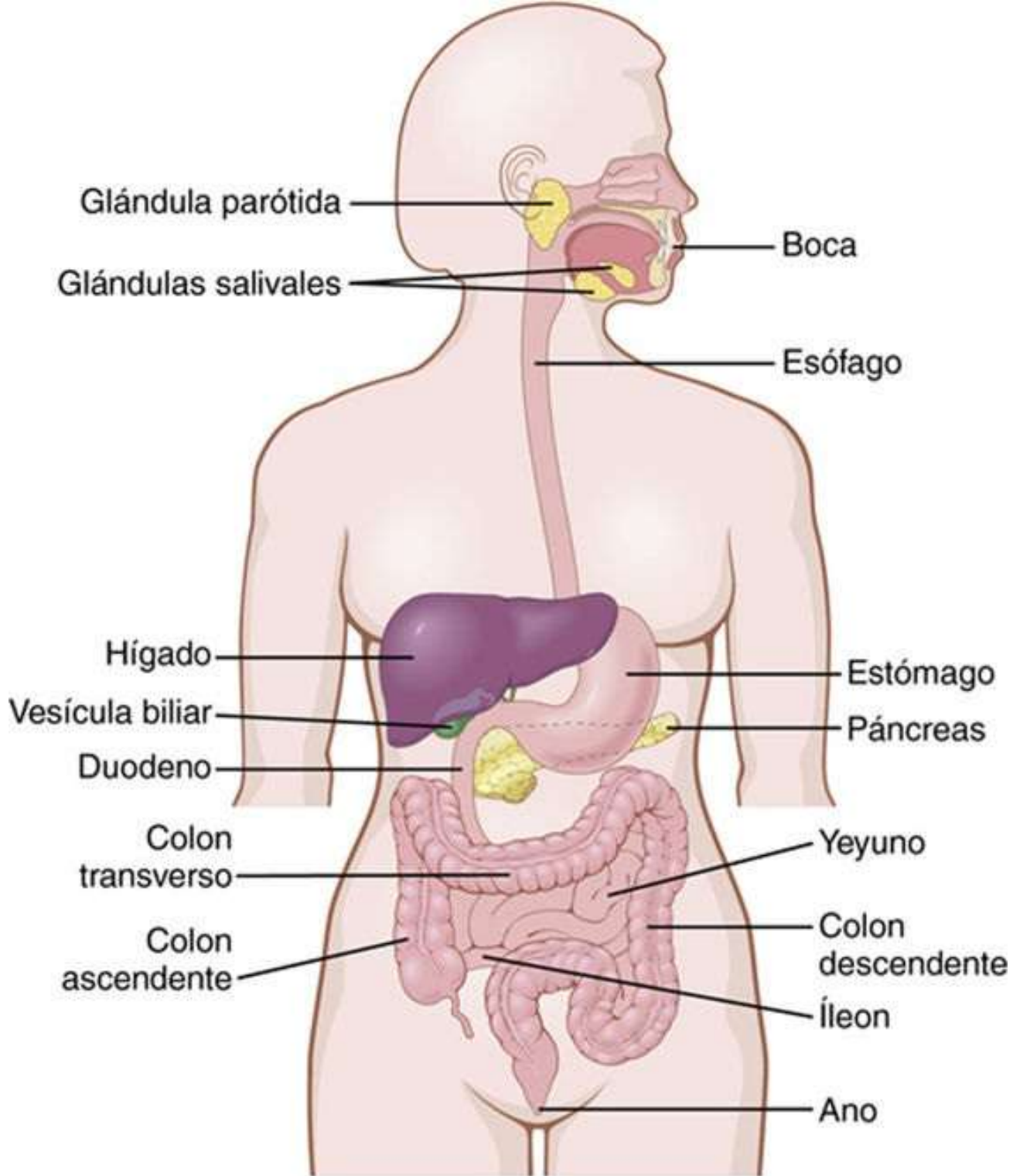
FIGURA 63-1 Aparato digestivo.
