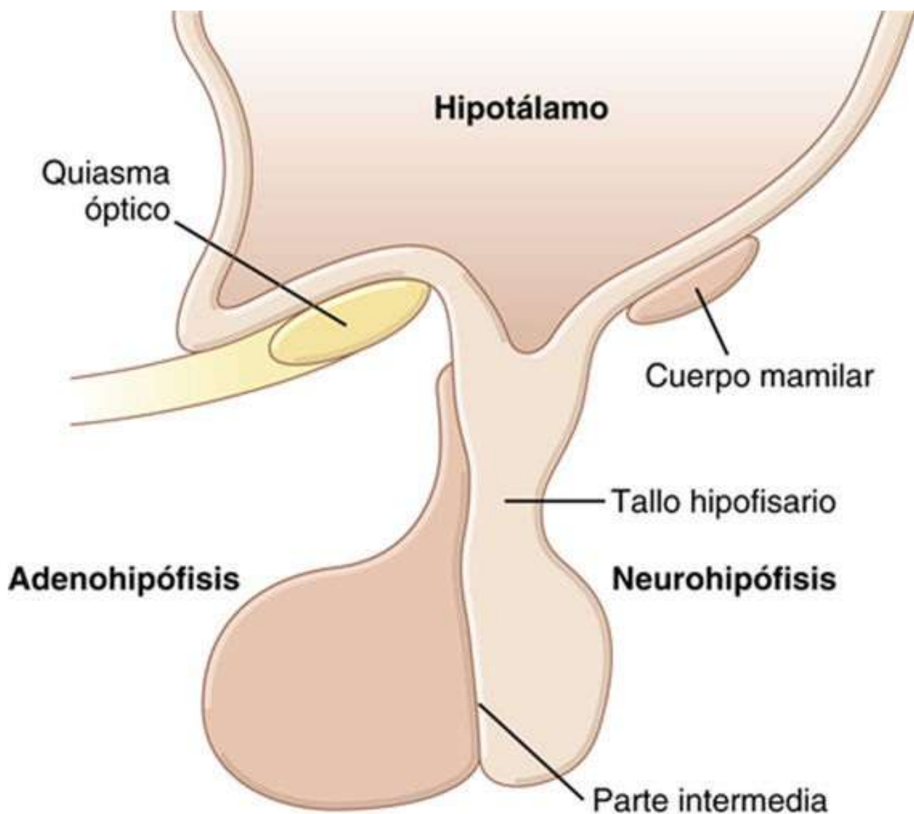
FIGURA 76-1 Hipófisis.
