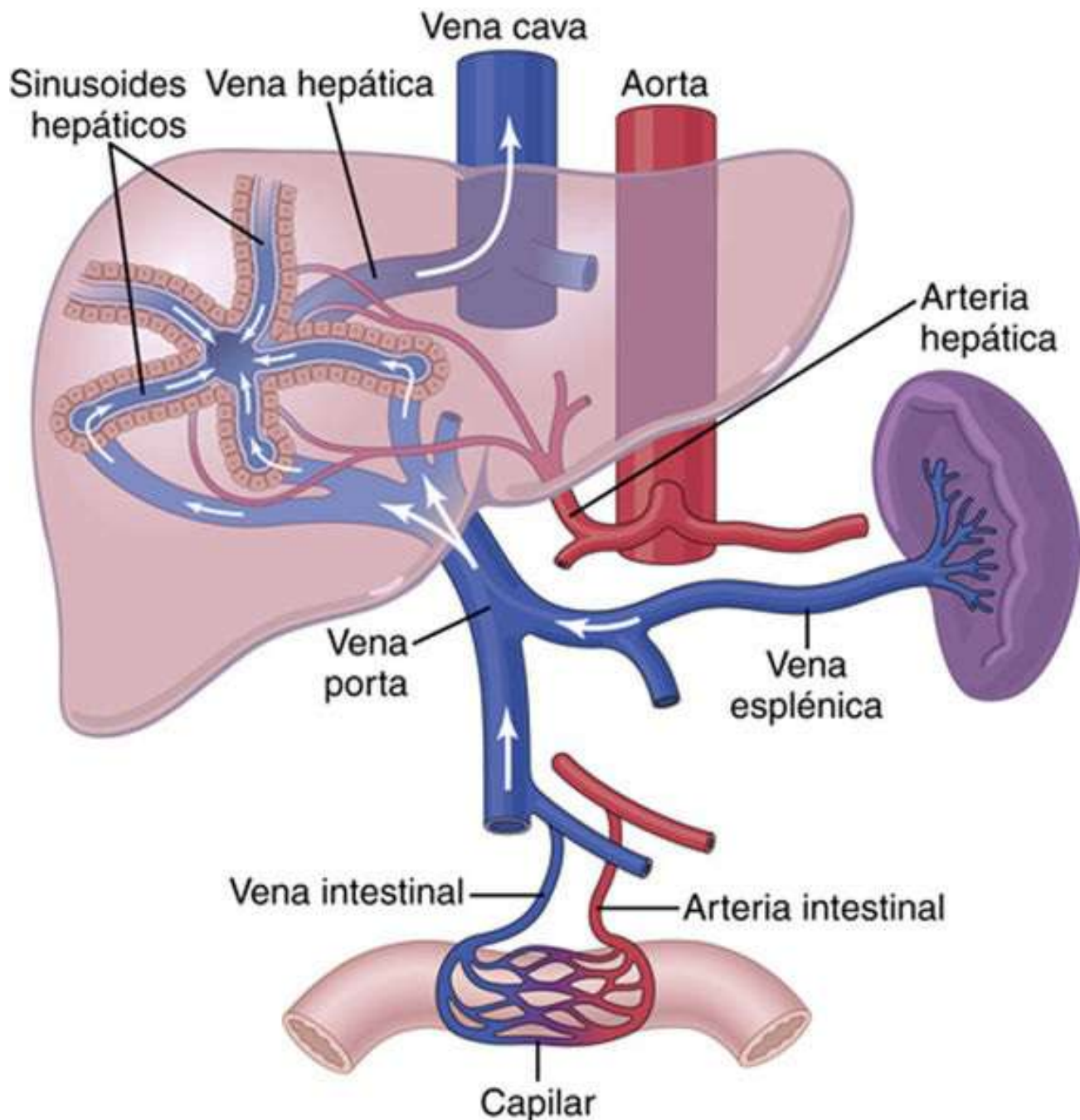
FIGURA 63-6 Circulación esplácica.
