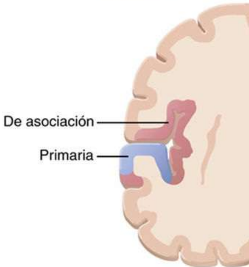
FIGURA 53-11 Corteza auditiva.
