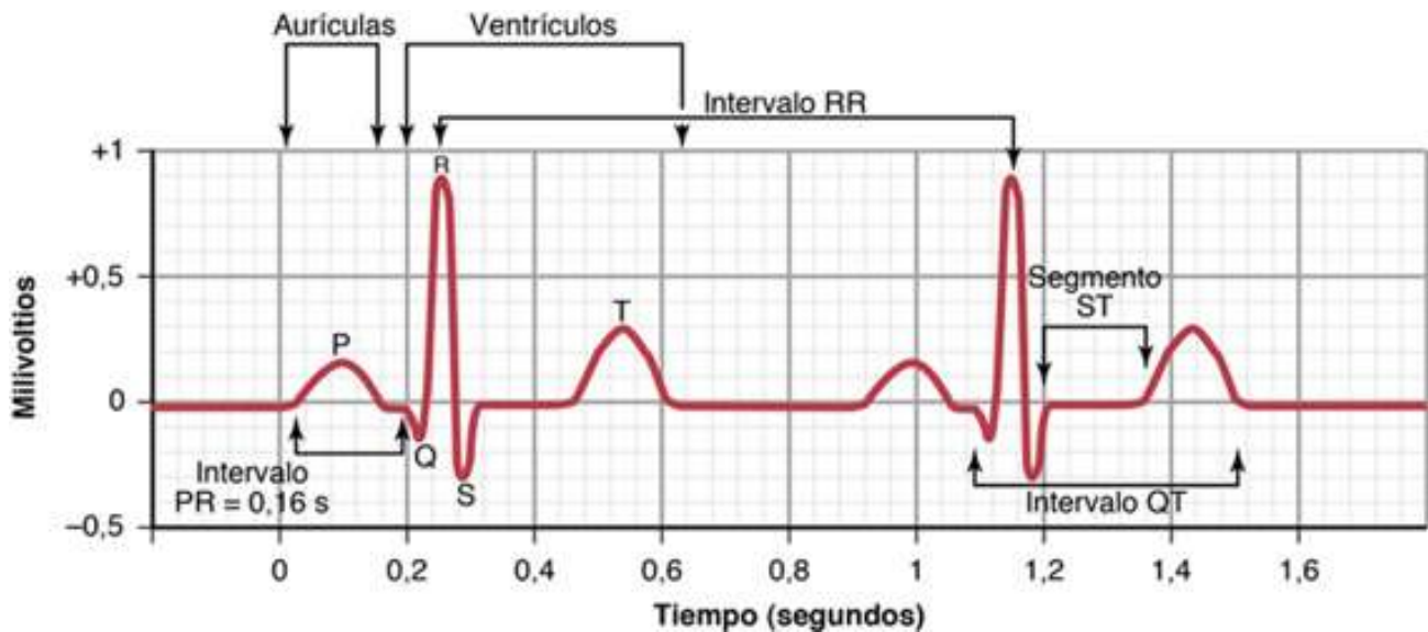
FIGURA 11-1 Electrocardiograma normal.
