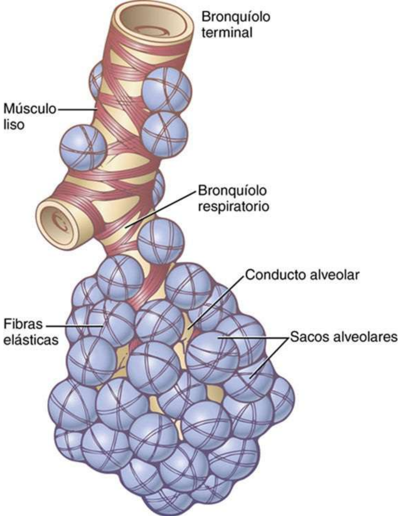
FIGURA40-7 Unidad respiratoria.
