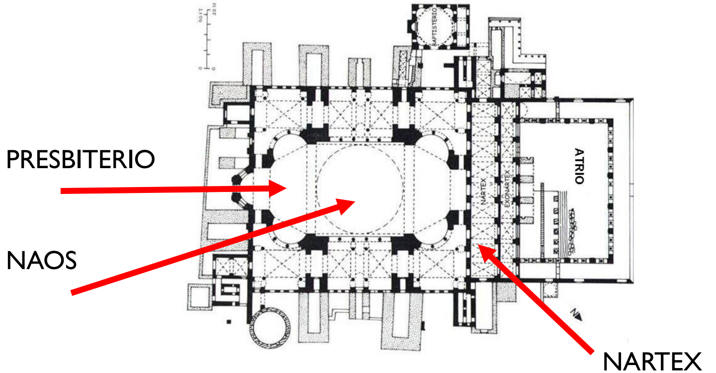
Basílica de Santa Sofía (532-537): planta de conjunto
