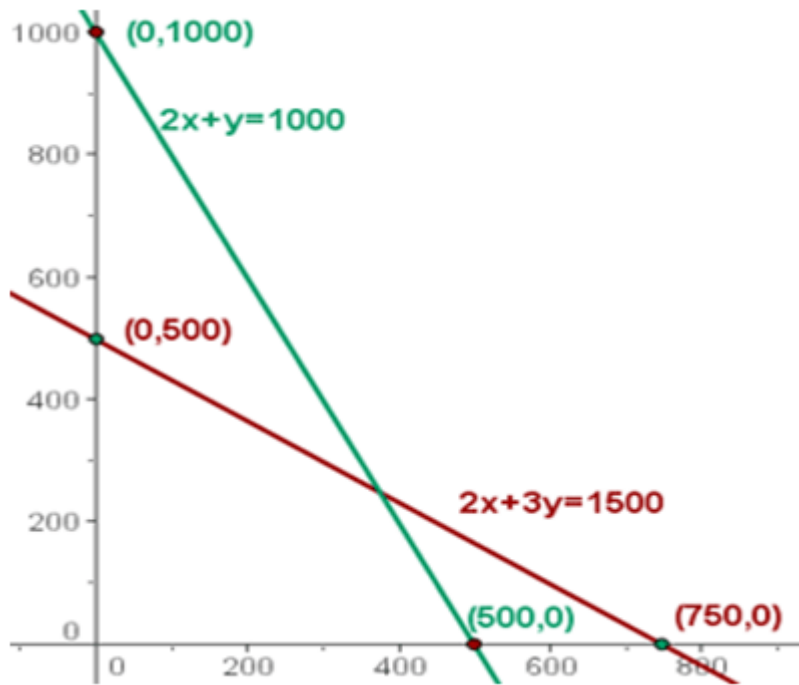
Programación lineal
